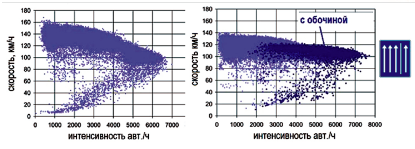
Рис. 4. Увеличение пропускной способности магистральной дороги – эффект применения временного снижения скорости до 120 км/ч и временного разрешения движения по обочине (Германия)
